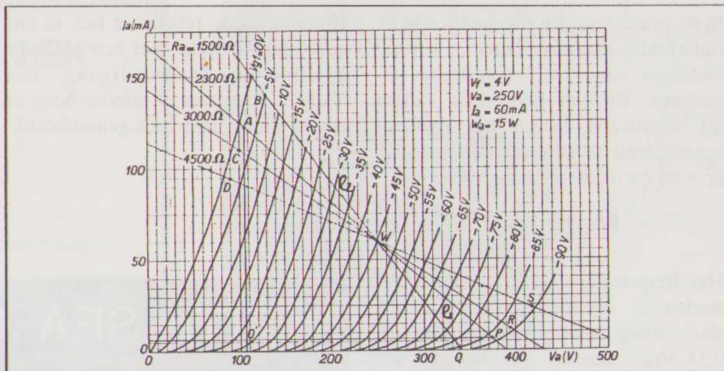
Fig. 2, karakteristiek I_a - V_g van een triode, waaruit de verhouding I1-I2 is af te leiden.
